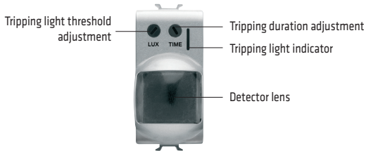
GW 10 591 - GW 12 591 - GW 14 591
