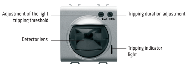
GW 10 592 - GW 12 592 - GW 14 592
