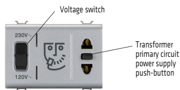
GW 10 331 - GW 12 331 - GW 14 331
