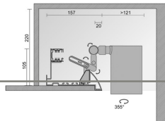
Sezione trasversale del sistema Broadway con proiettore Perfecto in posizione interna Cross section of Broadway system with Perfecto spotlight in internal position
