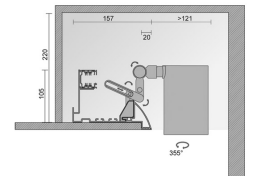
Sezione trasversale del sistema Broadway con proiettore Perfecto in posizione interna Cross section of Broadway system with Perfecto spotlight in internal position
