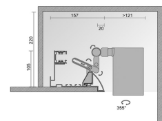
Sezione trasversale del sistema Broadway con proiettore Perfetto in posizione interna Cross section of Broadway system with Perfetto spotlight in internal position
