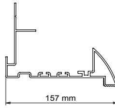
Art. 7840
