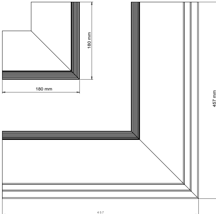
Art. 7850I
