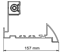
Art. 7841
