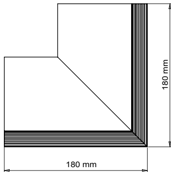
Art. 7850I
