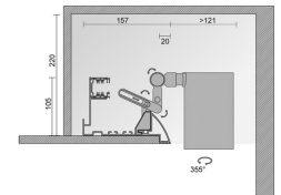
Sezione trasversale del sistema Broadway con proiettore Perfetto in posizione interna Cross section of Broadway system with Perfetto spotlight in internal position
