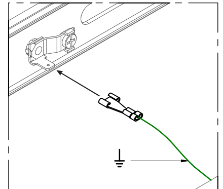
DETTAGLIO B
