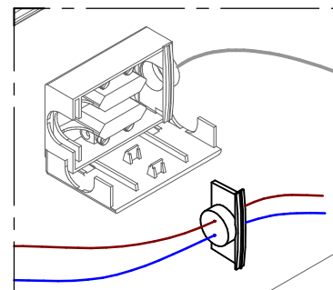
DETTAGLIO A
