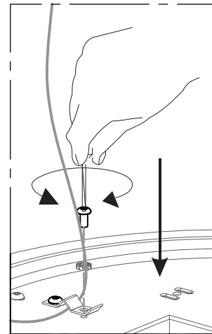
DETTAGLIO B
