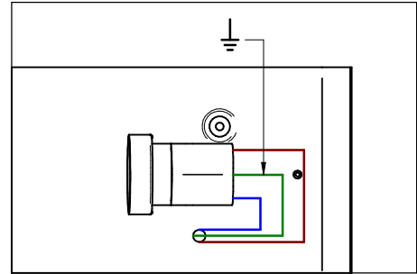
DETTAGLIO CABLAGGIO
